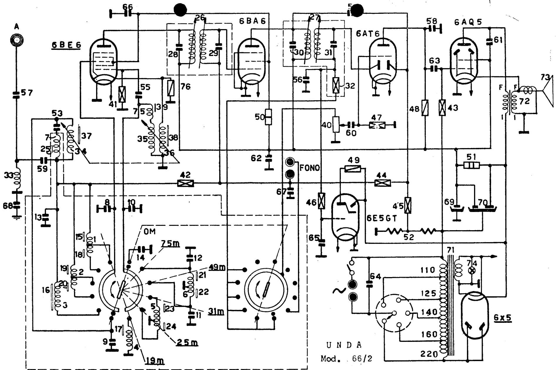
UNDA RADIO - Mod. R 66/2. Ricevitore con sintonia a permeabilità variabile. Una gamma onde medie e cinque bande allargate ad onde corte. Media frequenza 467 kc/s. Potenza indistorta di uscita 3 watt. Consumo 35 watt. (V. a parte tabella valori).
